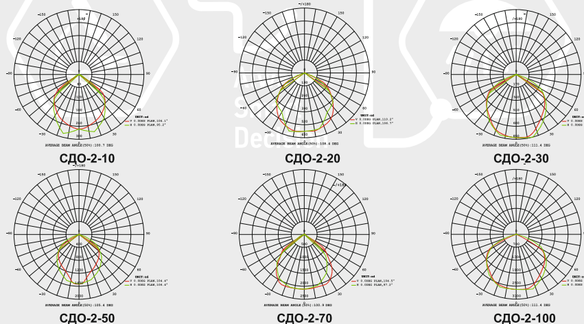
Рис. 1. Кривые силы света
